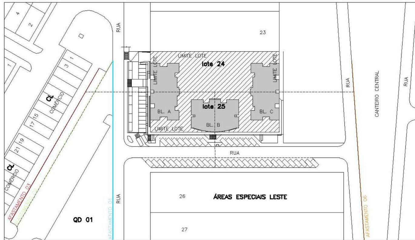
PLANTA DE SITUAÇÃO e LOCAÇÃO
